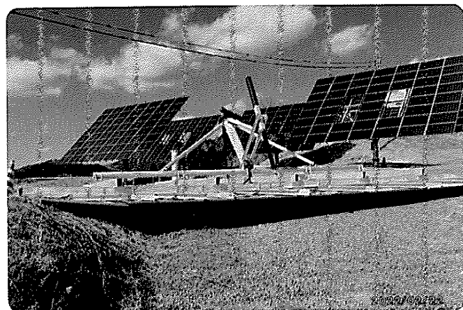
▲ 倒壊した太陽光発電
