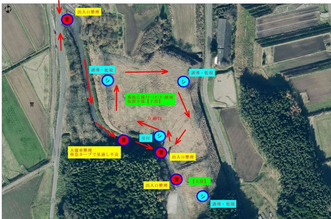
交通誘導員 配置図
