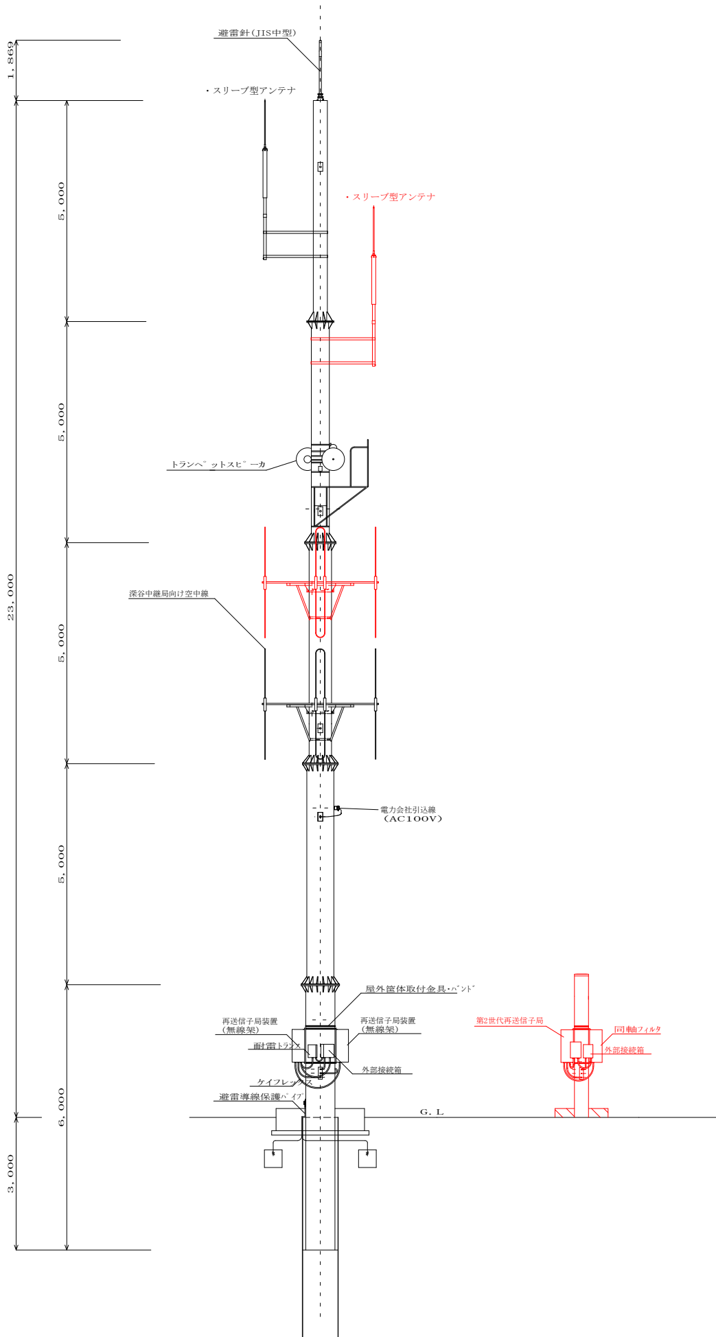
永山再送信局空中線柱装柱図 (地上高23m)
