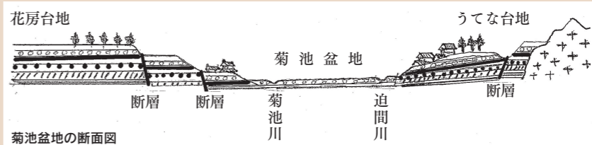
菊池盆地の断面図
